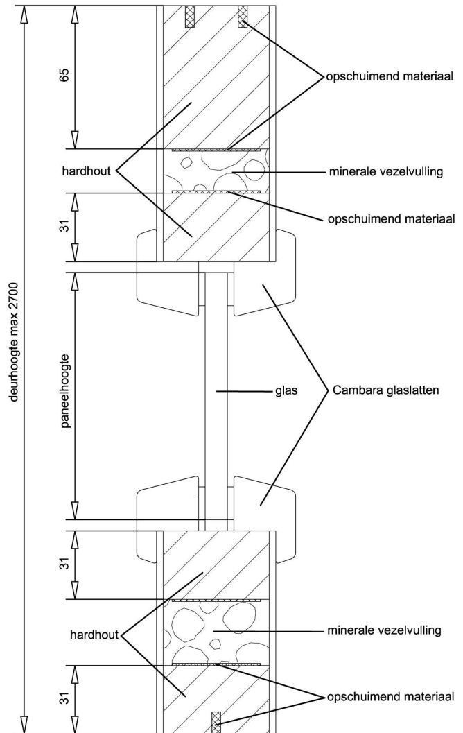
Doorsnede BB
