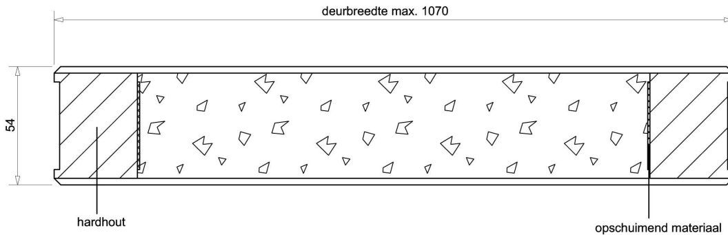
Doorsnede AA
