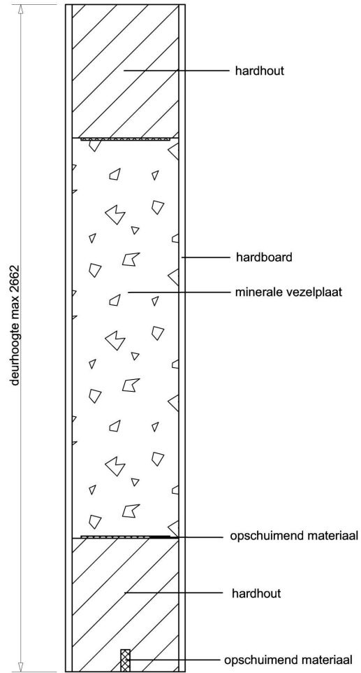
Doorsnede BB
