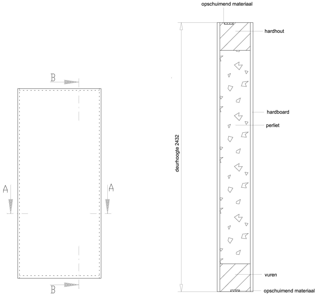
Doorsnede BB
