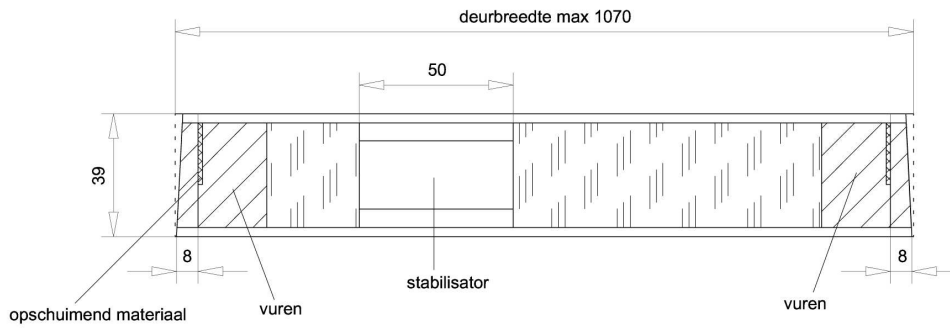
Doorsnede AA
