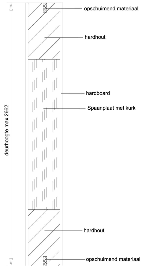
Doorsnede BB
